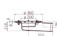
van gietijzer met klemflens met sijpelopeningen zijuitlaat gewicht ca. 15,2 kg
